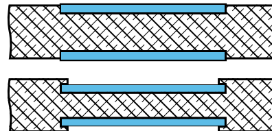
ДВА СКЛА ПО 4 ММ
