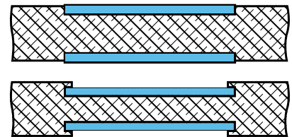
ДВА СКЛА ПО 4 ММ
